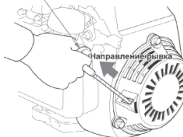
РУКОЯТЬ СТАРТЕРА
